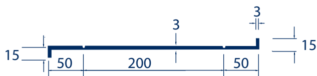
Aleta 3 mm
