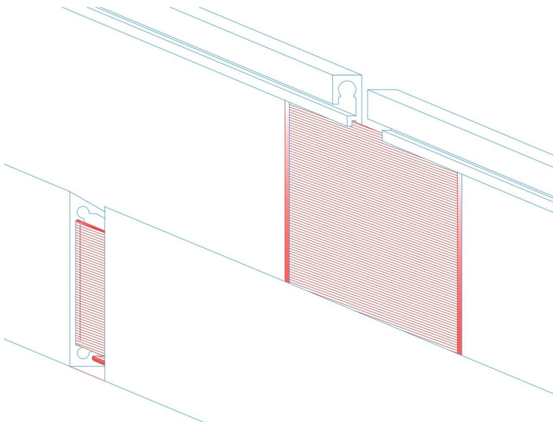
Ligação entre dois perfil viga-calha
